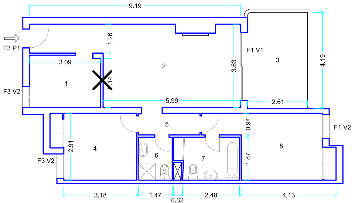
PLANTA BAJA
